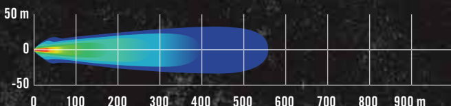
10" OnX6 Combo
